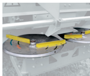
Разбрасывающие тарелки и лопатки из нержавеющей стали (ширина распределения 24-36 м)
